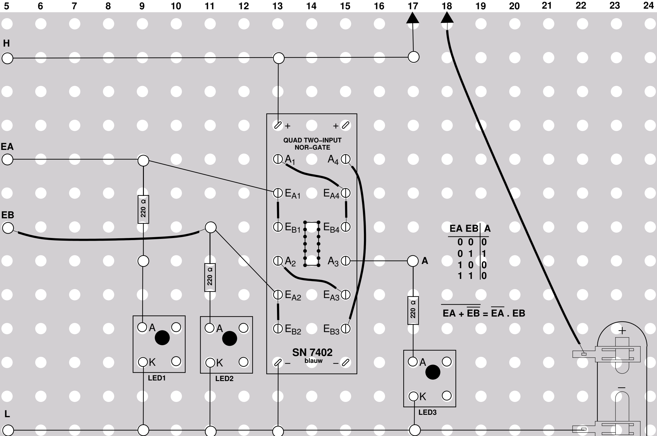
4.10.14. AND met een inverterende ingang
